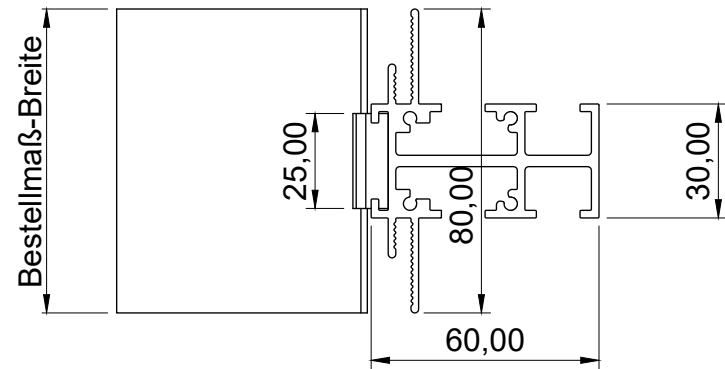
Draufsicht
