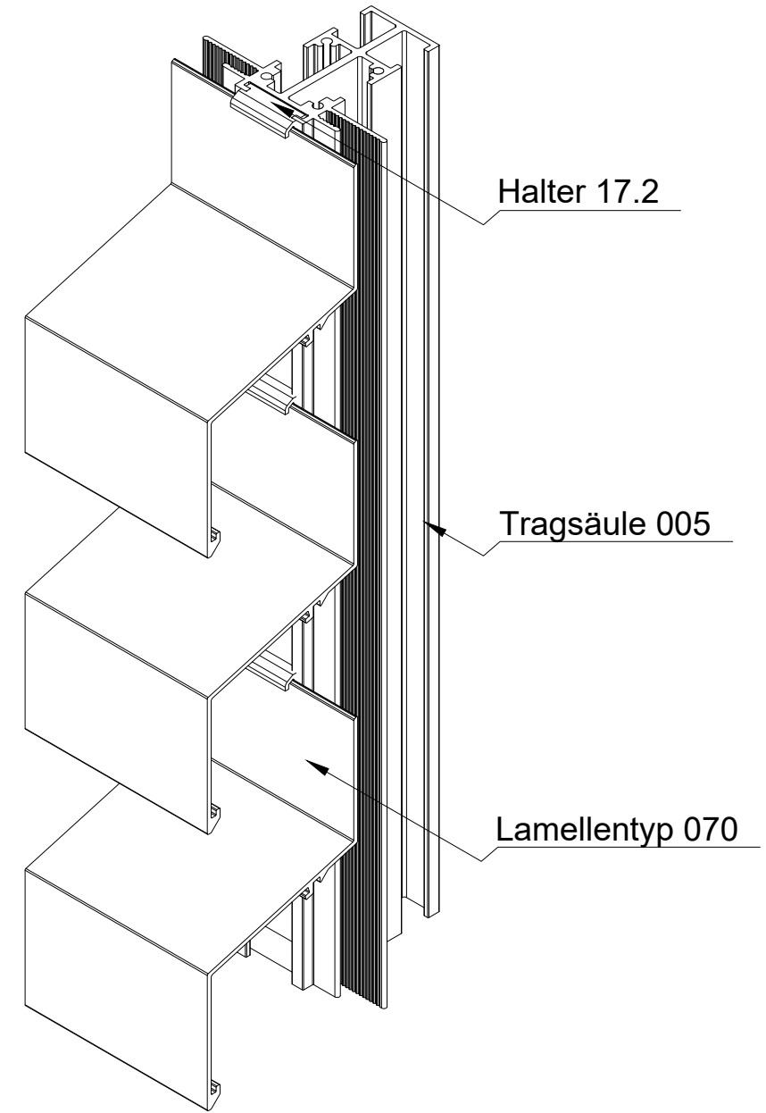
ISO-Ansicht
