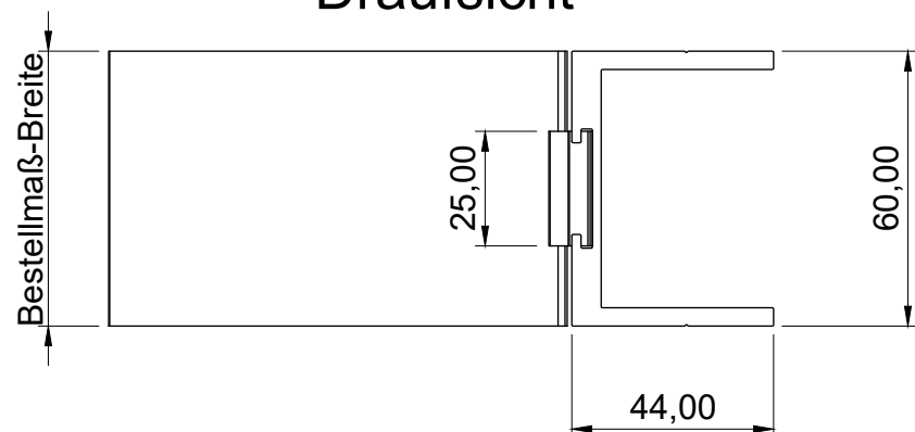
Draufsicht
