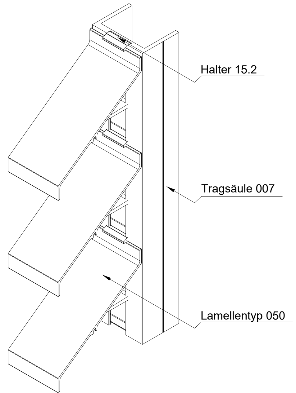
ISO-Ansicht
