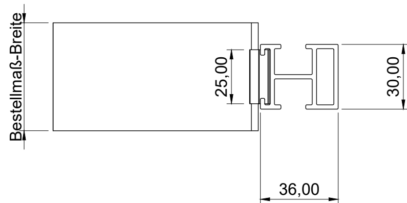
Draufsicht
