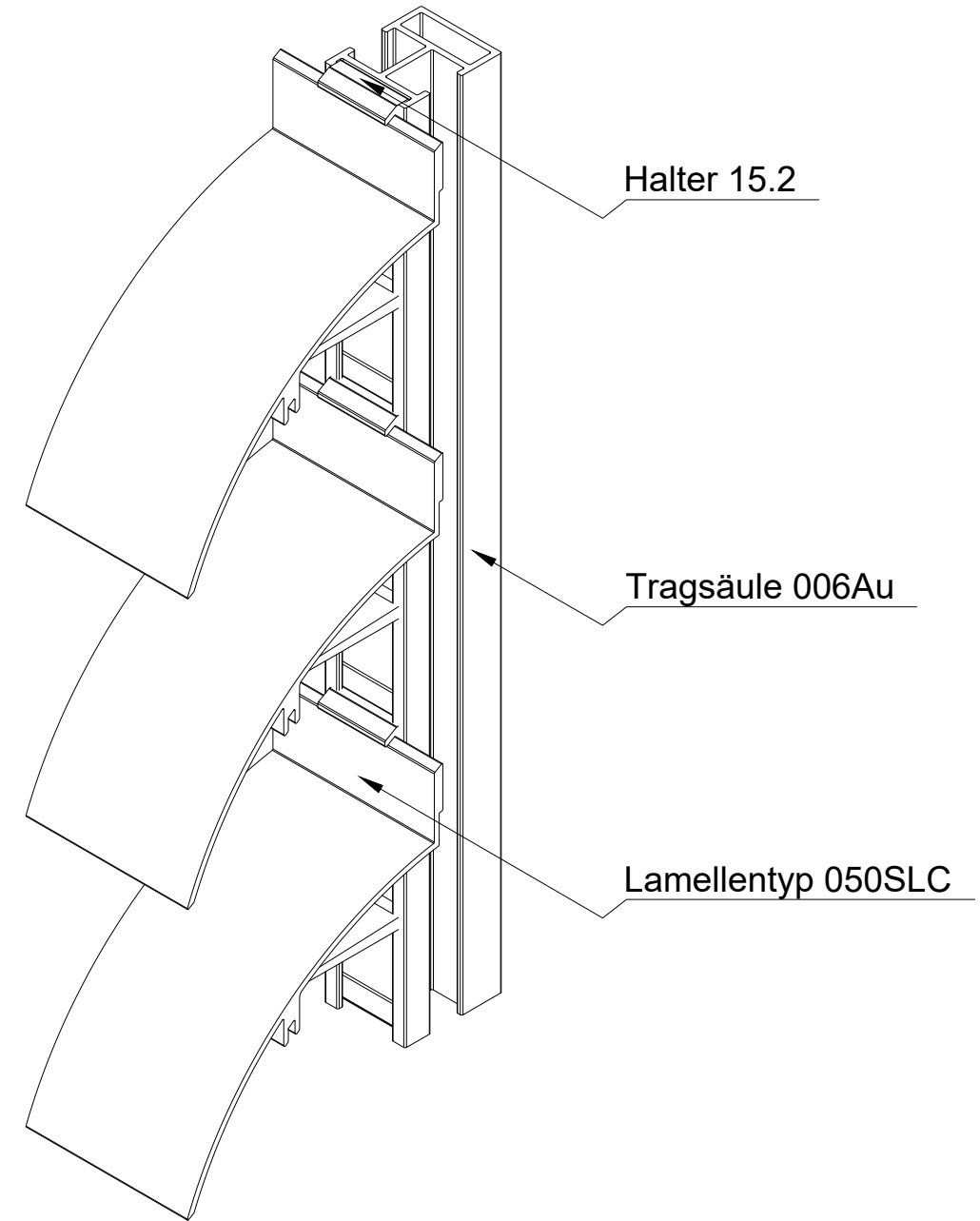
ISO-Ansicht
