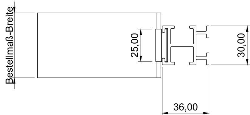
Draufsicht
