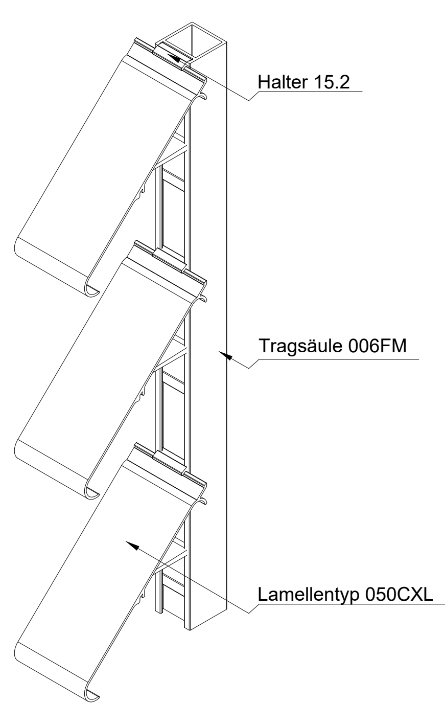
ISO-Ansicht
