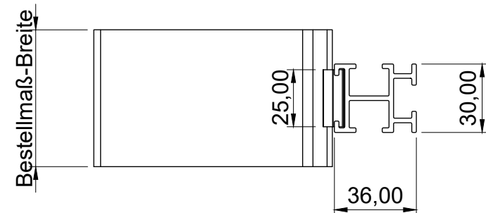
Draufsicht
