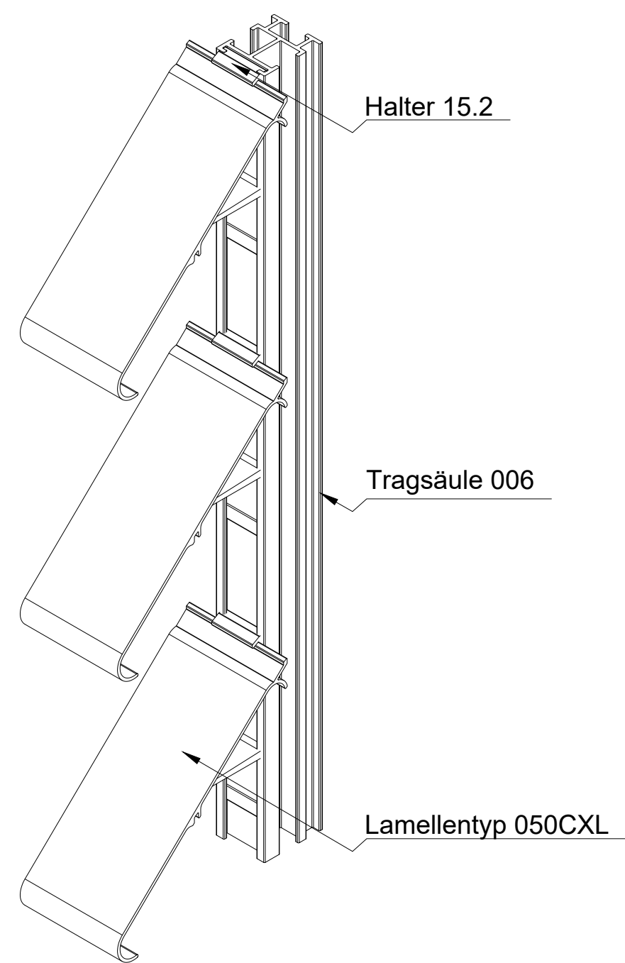
ISO-Ansicht
