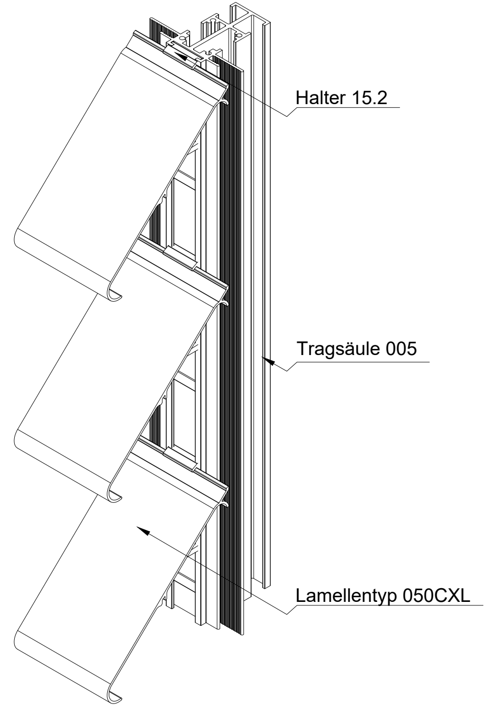
ISO-Ansicht
