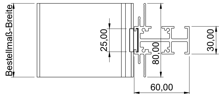
Draufsicht
