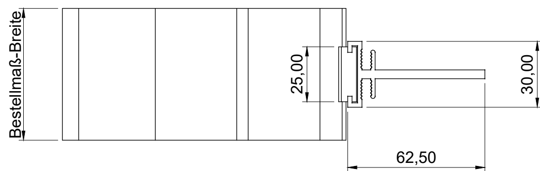
Draufsicht
