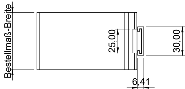
Draufsicht
