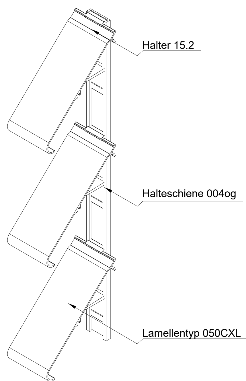
ISO-Ansicht
