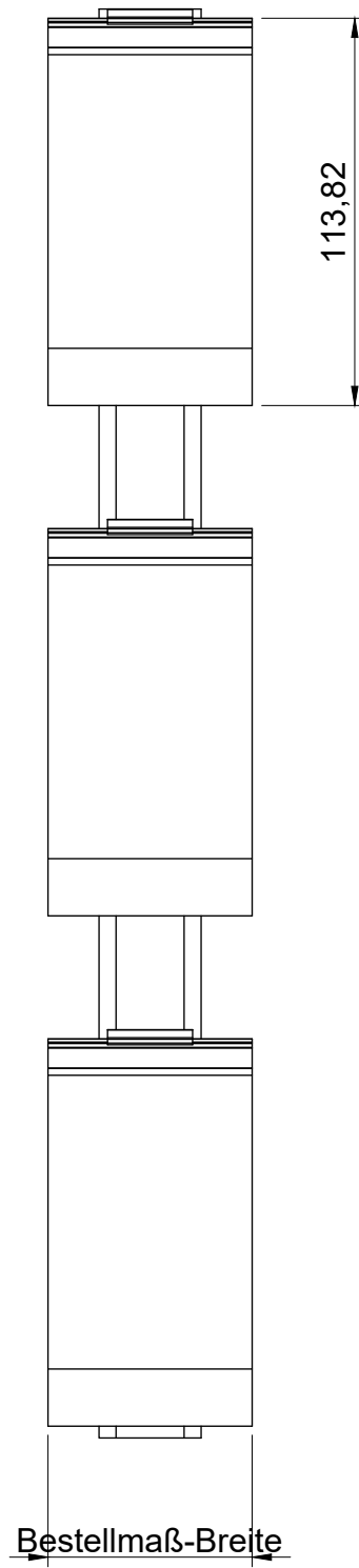
Seitenansicht
