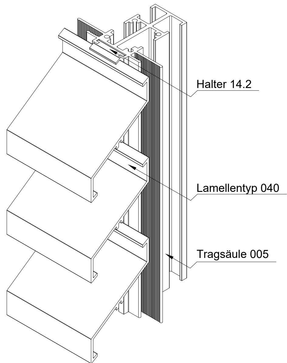
ISO-Ansicht
