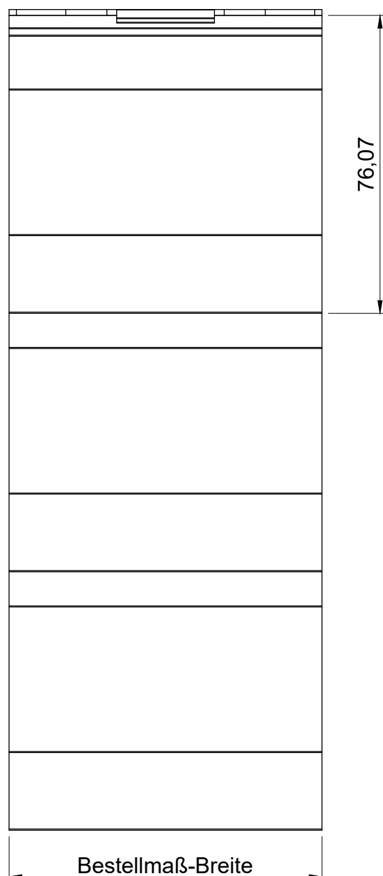
Seitenansicht
