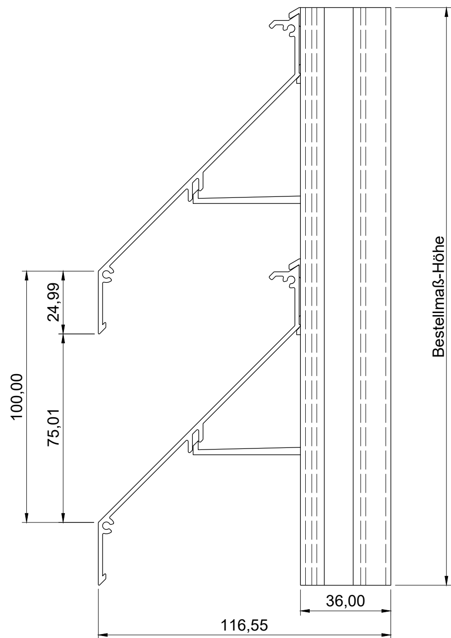
Draufsicht
