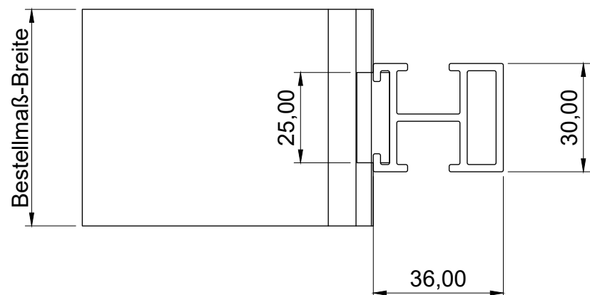
Draufsicht
