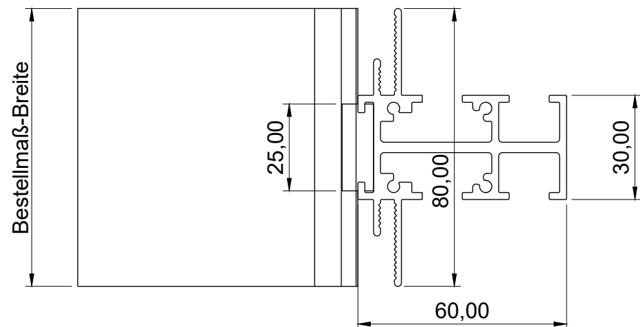
Draufsicht
