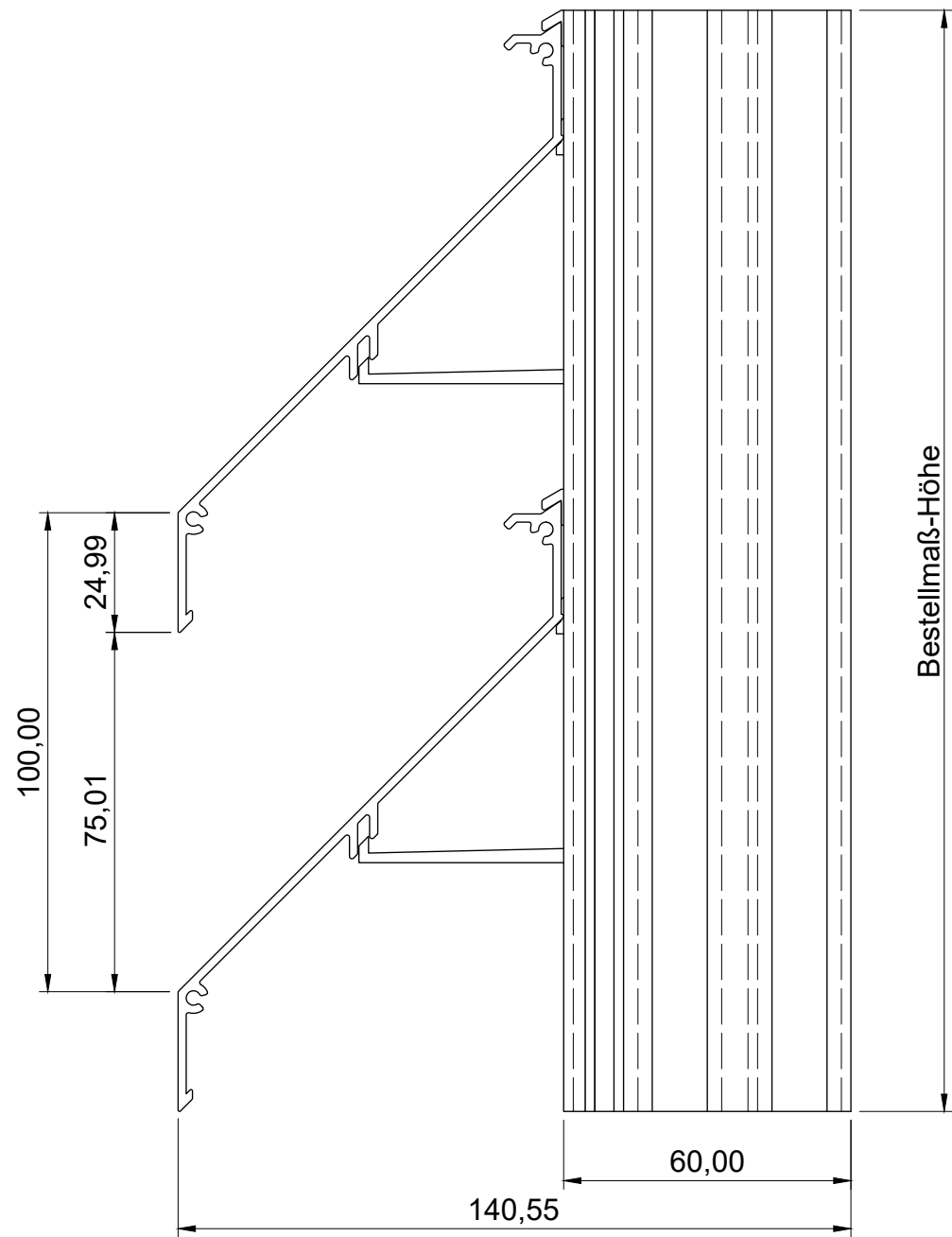
Draufsicht
