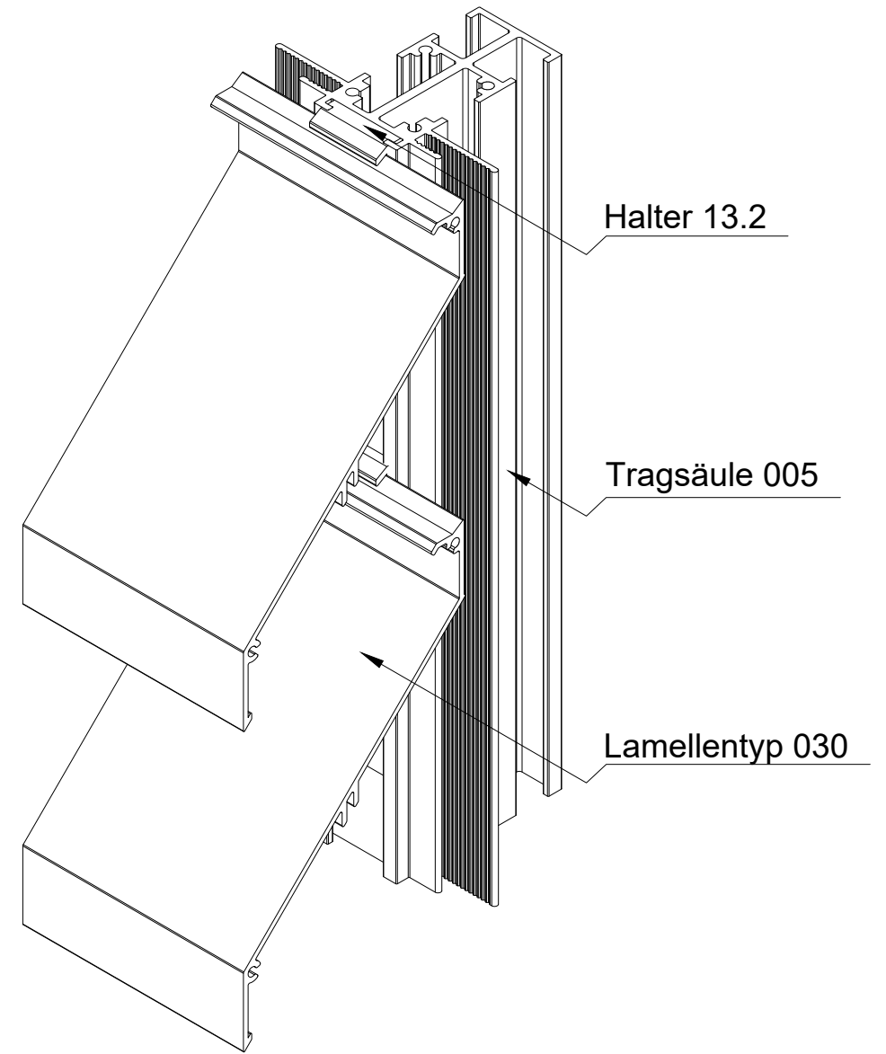
ISO-Ansicht
