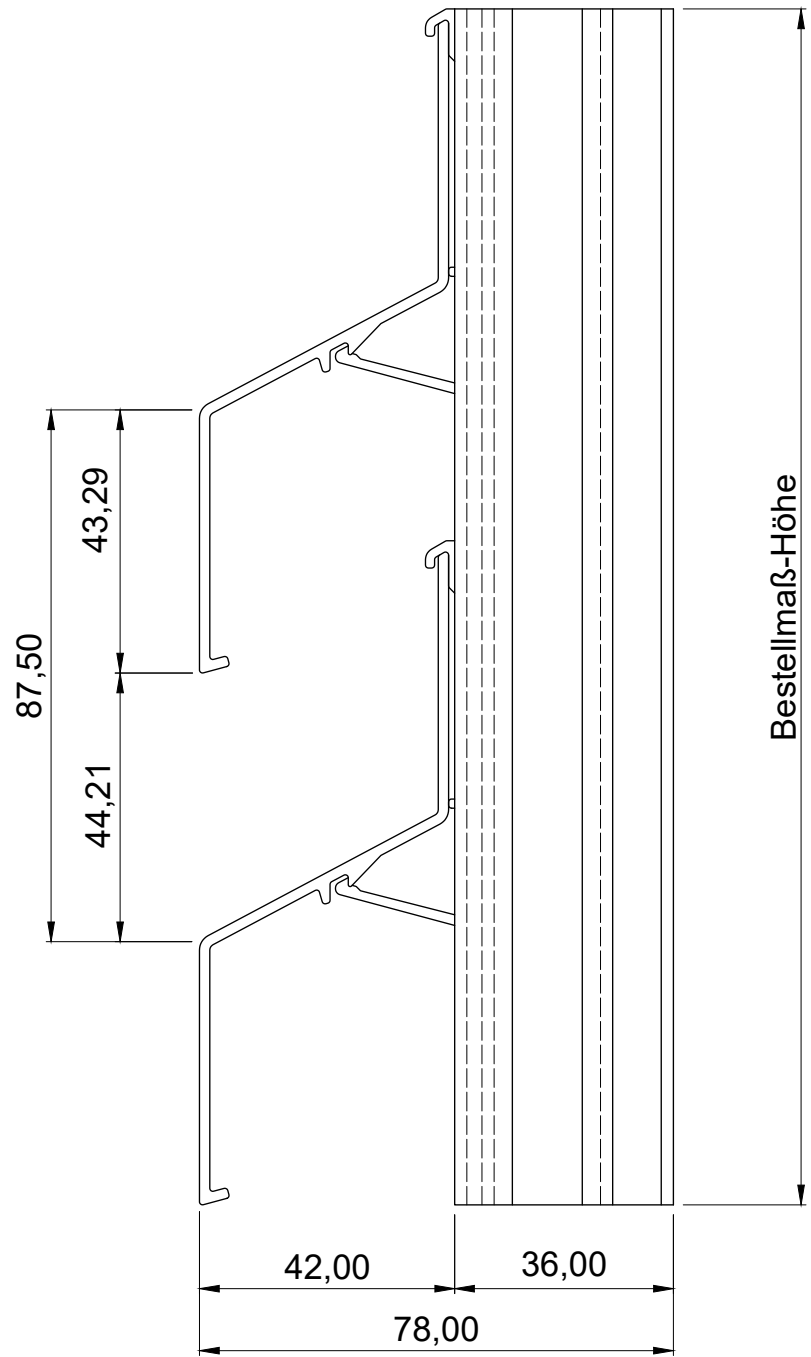
Vorderansicht
