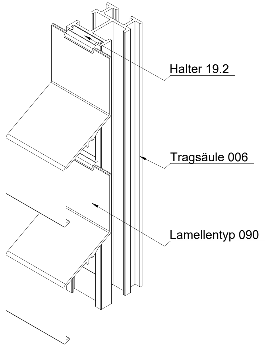
ISO-Ansicht
