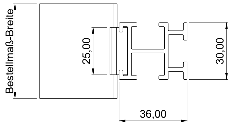
Draufsicht
