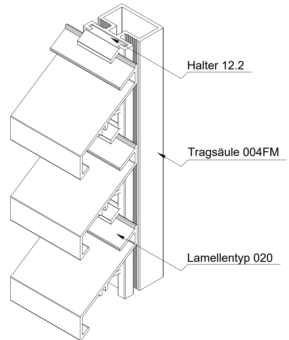
ISO-Ansicht
