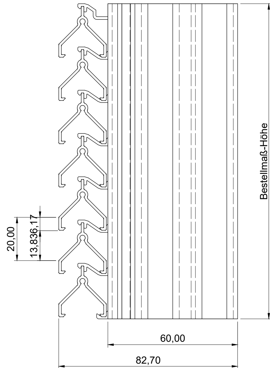
Draufsicht
