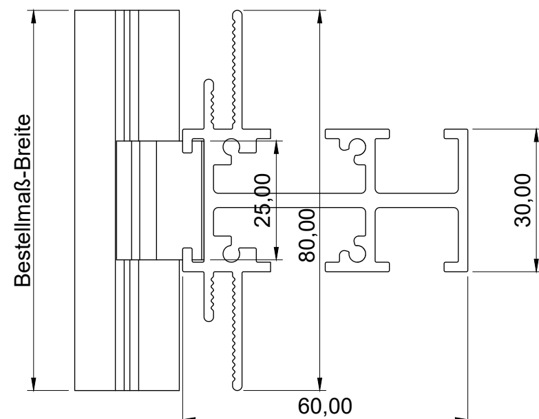
Draufsicht
