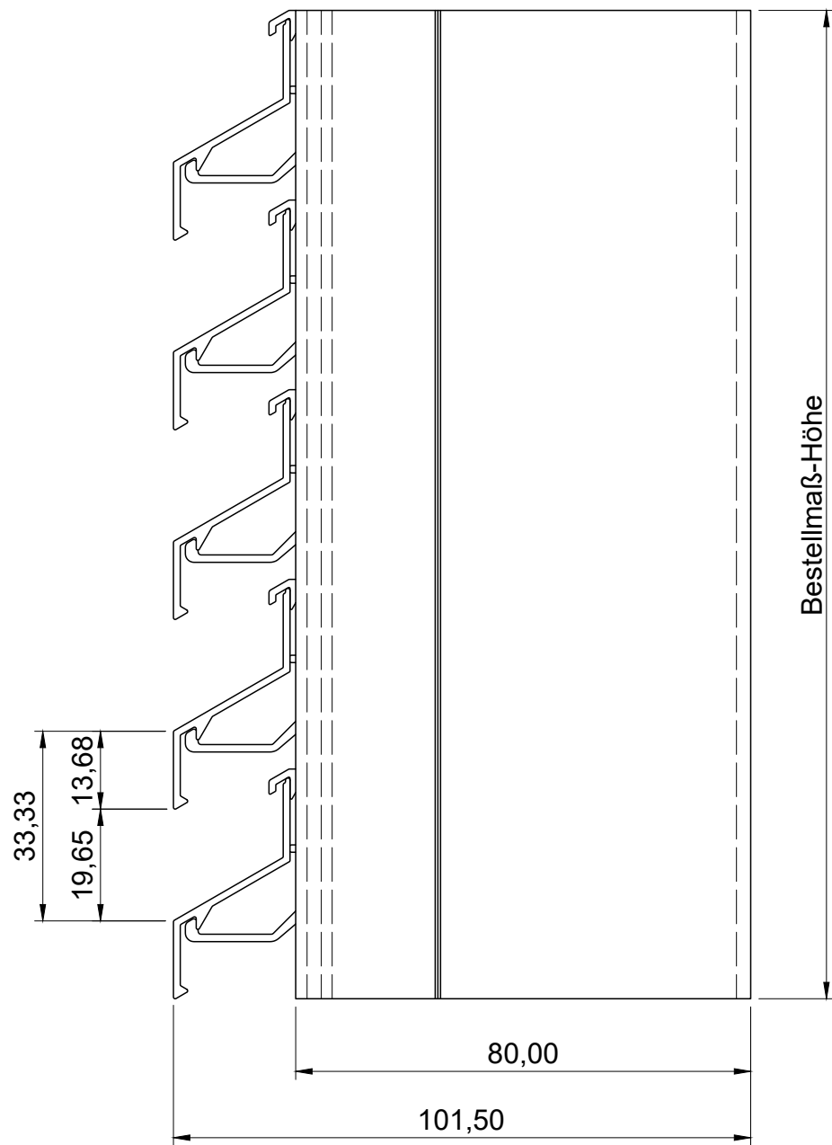
Draufsicht
