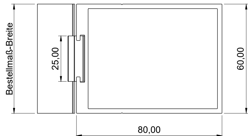
Draufsicht
