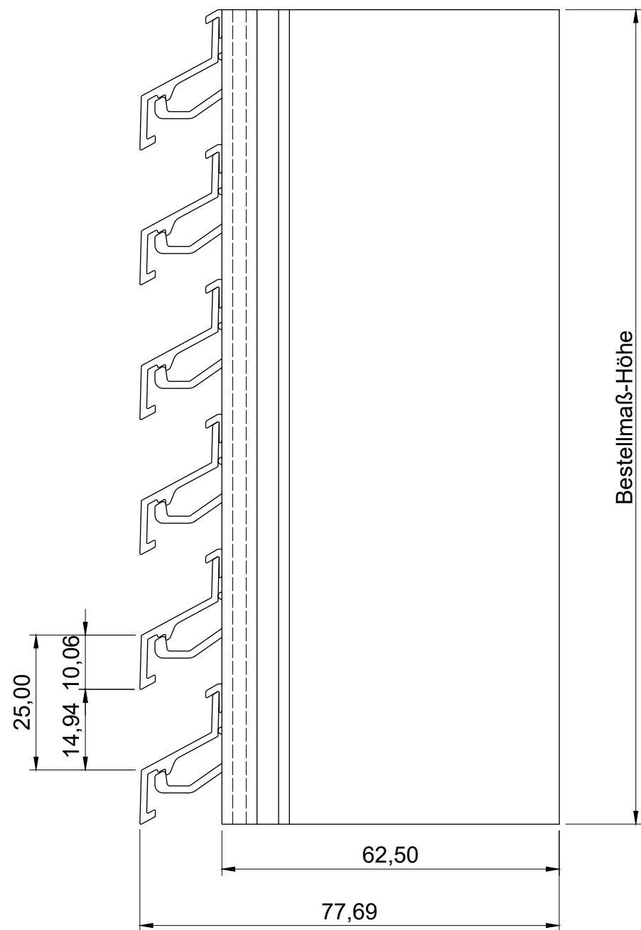
Draufsicht
