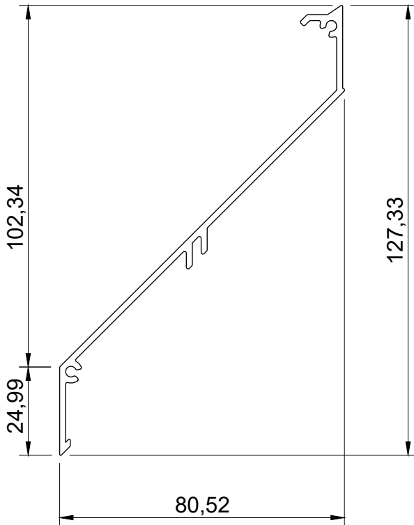
Vorderansicht
