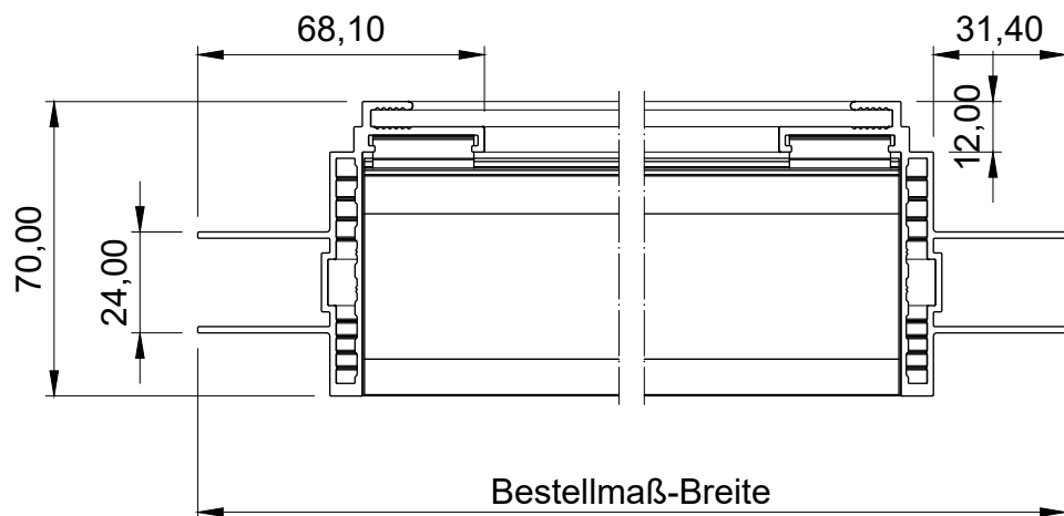
Draufsicht
