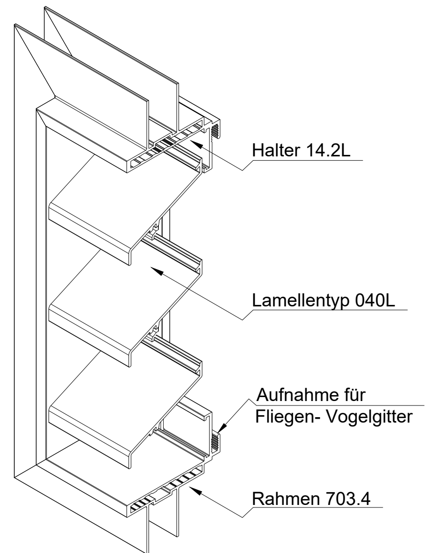
ISO-Ansicht
