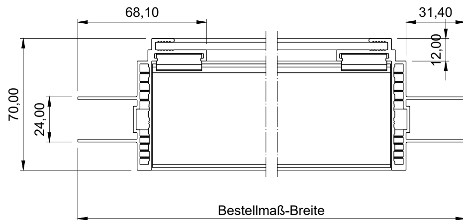
Draufsicht
