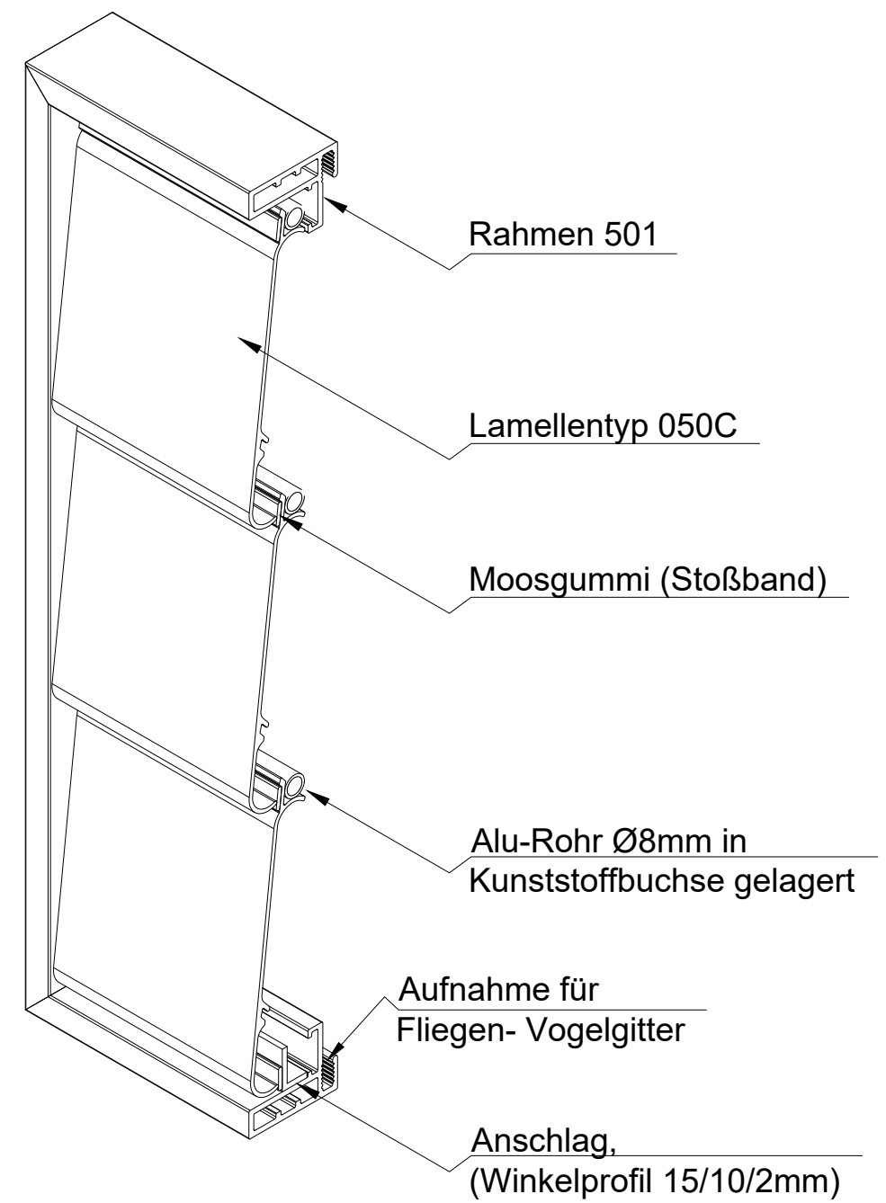
ISO-Ansicht
